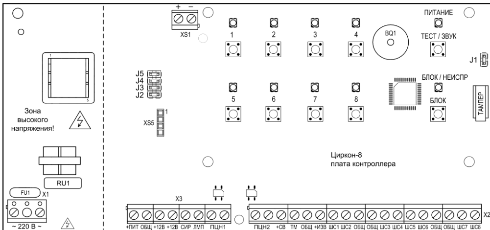
Рис.1 Плата контроллера прибора
