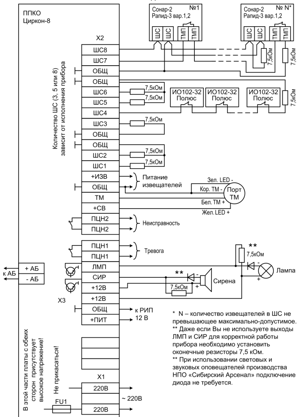
Рис.А1 Схема внешних соединений ППКО Циркон-8
