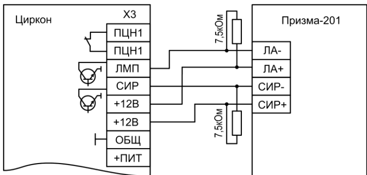
Рис.А2 Схема подключения оповещателя свето-звучового «Призма-201»
