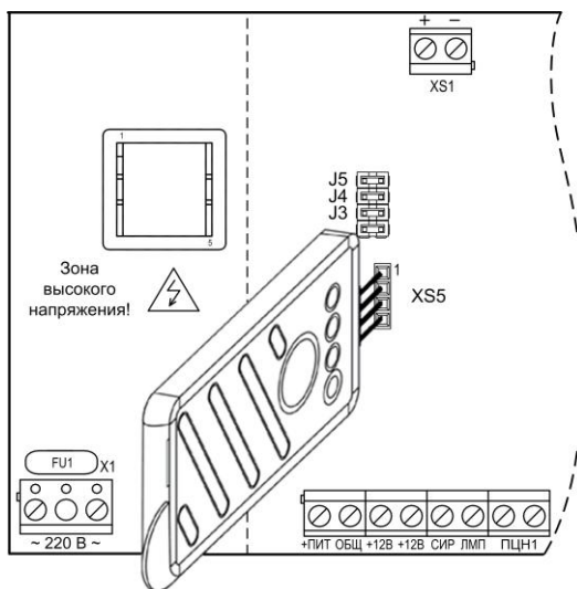
Рис.А3 Подключение USB-программатора к плате ППКО Циркон
